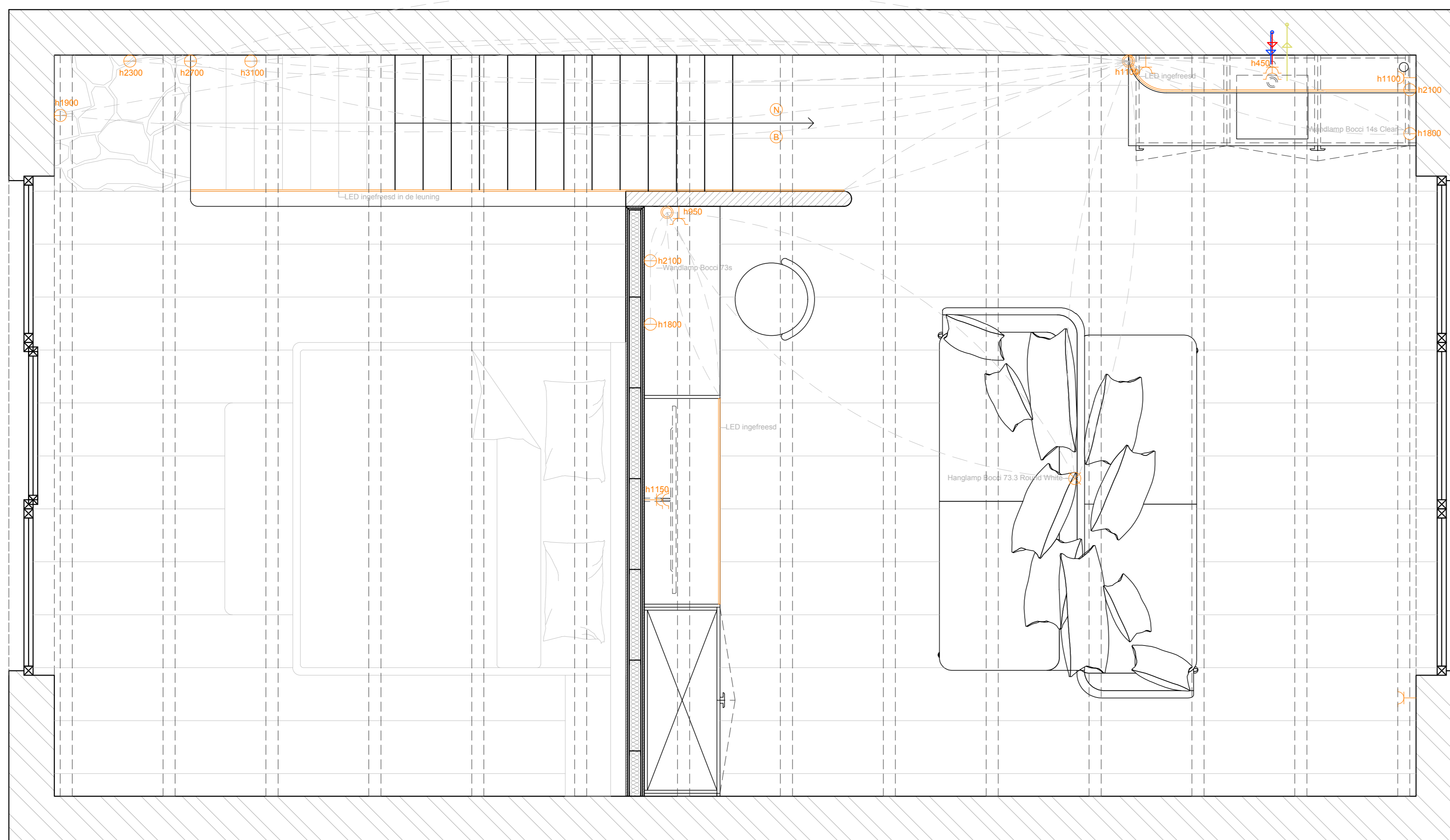
TECHNISCH PLAN EERSTE VERDIEP (sanitair + elektriciteit) 1:20
