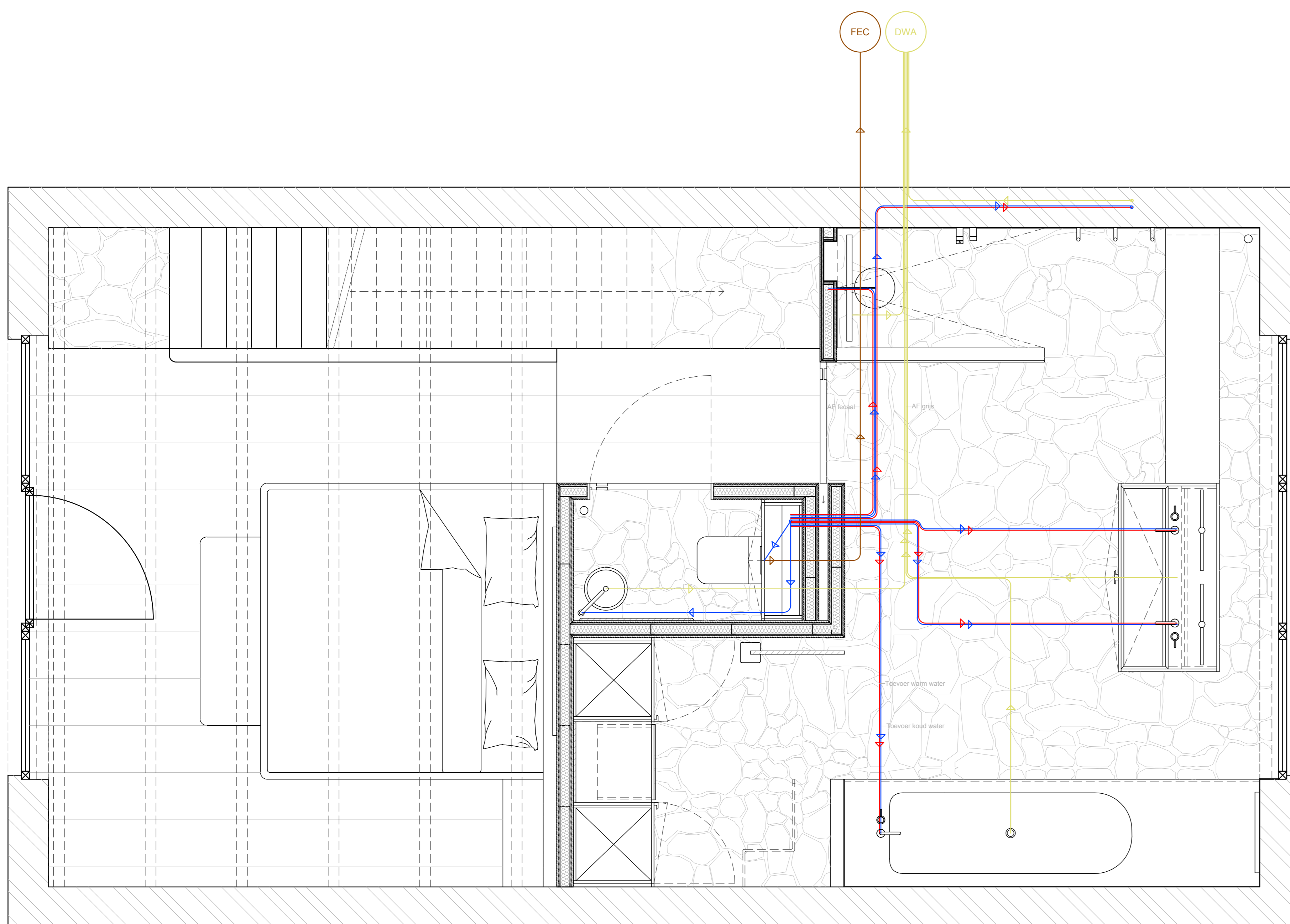
TECHNISCH PLAN GELUKVLOERS (sanitair) 1:20
